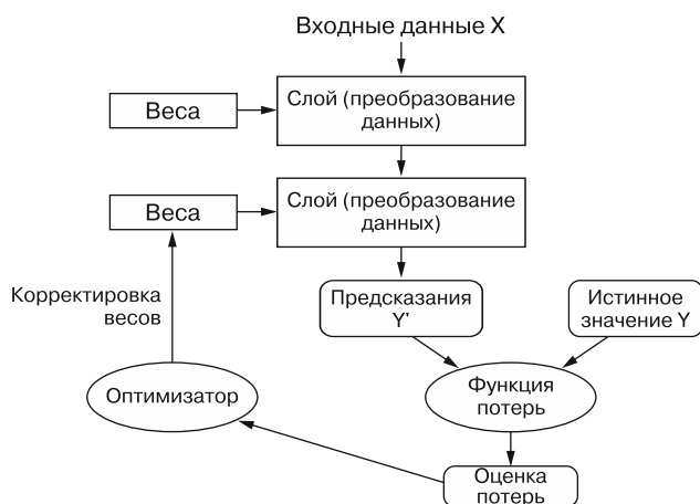
Рис. 1.9. Оценка потерь используется как обратная связь для корректировки весов
