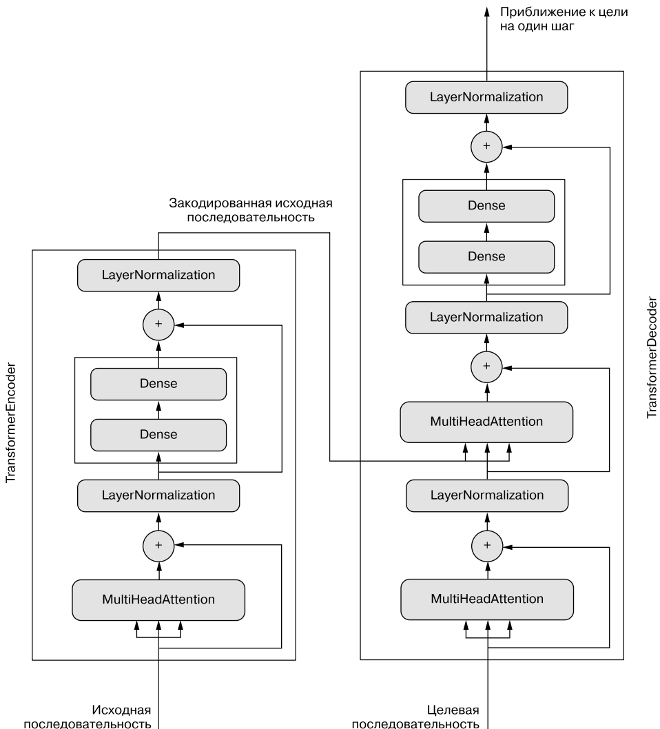
Рис. 11.14. TransformerDecoder похож на TransformerEncoder , за исключением дополнительного блока внимания, где ключи и значения представляют исходную последовательность, закодированную с помощью TransformerEncoder . Вместе кодировщик и декодер образуют сквозную модель Transformer
