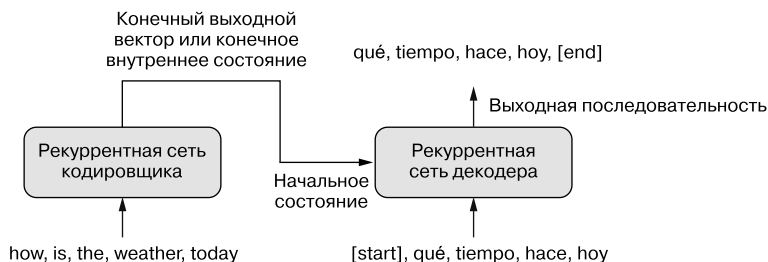
Рис. 11.13. Рекуррентная модель типа «последовательность в последовательность»: рекуррентная сеть кодировщика создает вектор, кодирующий всю исходную последовательность, а далее этот вектор используется в качестве начального состояния рекуррентной сети декодера
