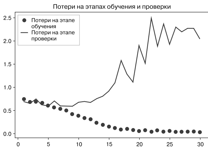
Рис. 8.9. Графики изменения метрик на этапе проверки при обучении простой сверточной сети
